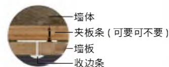
@顶视剖面图
