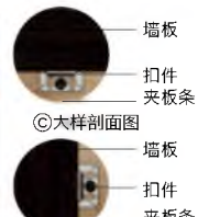
③大样剖面图
